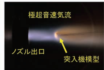
アーク風洞による大気圏突入実験
